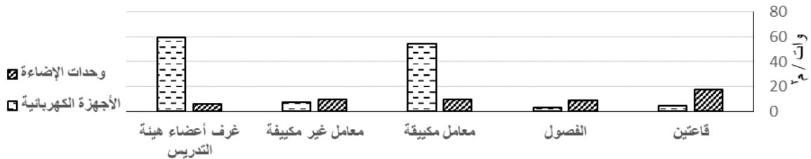
شكل ٢١: يوضح معدلات استهلاك الطاقة لوحدة الإضاءة والأجهزة المختلفة في الدور الثالث علوى
