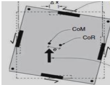
الشكل (2): تشكل عزم قتل [1]
