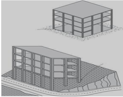
الشكل (12): حالات تشكل الأعمدة القصيرة. [1]
