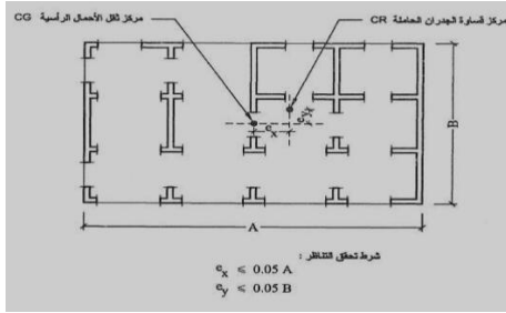
الشكل (1): التناظر الإنشائي في المسقط الأفقي [9]
