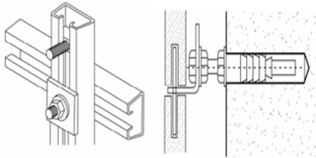
الشكل(7): طريقة تثبيت العناصر غير الإنشائية [3]
