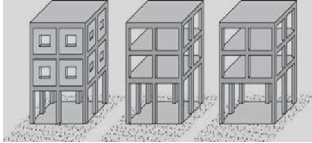
الشكل (11): الاستمرار بالعناصر الإنشائية يجنب المبنى عزم الفتل [5]
