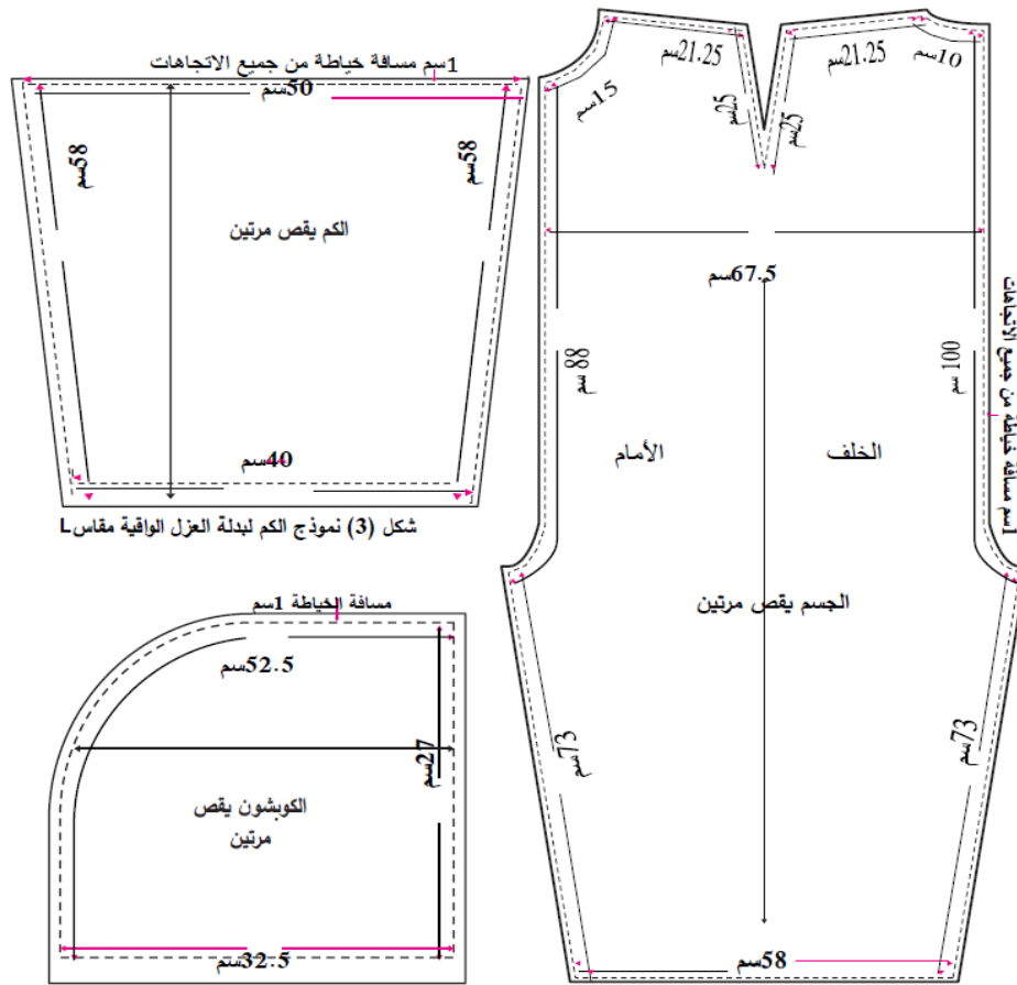
شكل (2) نموذج الجسم (أمام وخلف) لبدة العزل الواقية مقاس L شكل (4) نموذج غطاء الرأس لبدة العزل الواقية مقاس L
