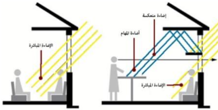
الشكل (6) توزيع الإنارة الطبيعية باستخدام الكاسرات.
