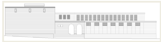
الشكل (23): الواجهة الشرقية لمتحف دمشق والتي تشبه واجهة الدخول بأسلوب الفتح. المصدر (المديرية العامة للآثار والمتاحف وعمل الباحث ) نفوذية الإنارة الطبيعية:
